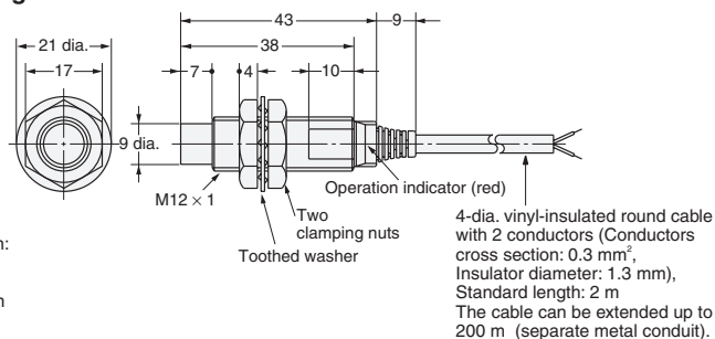
Fig. 11: E2E-X5MY
