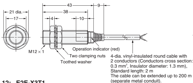
Fig. 12: E2E-X3T1
